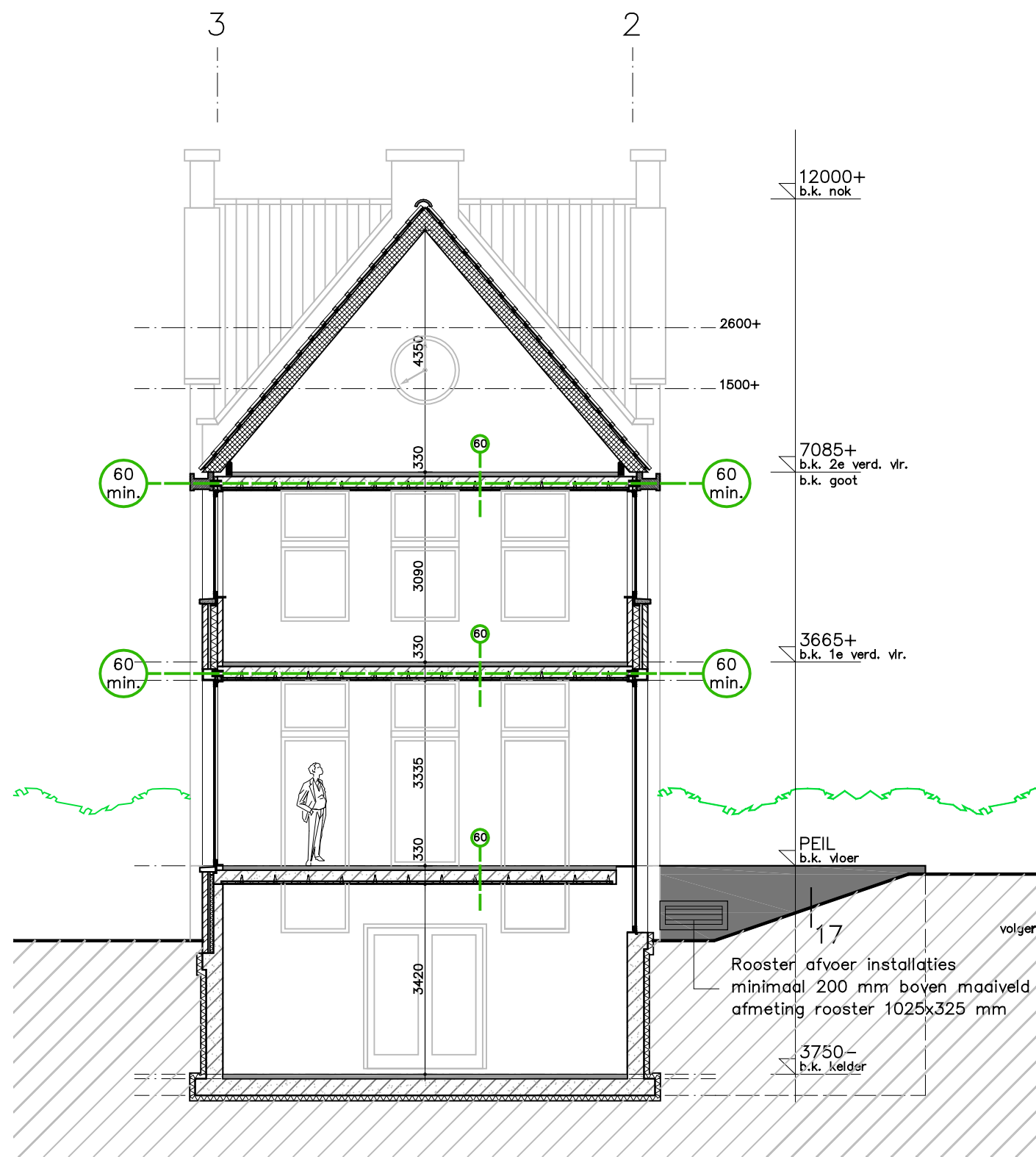
DOORSNEDE A-A
